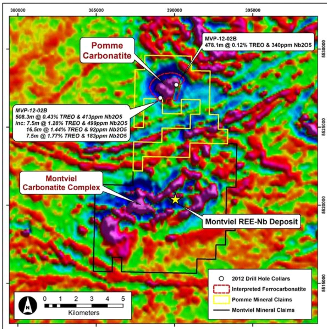
Figure 1 : Image magnétique aéroportée du projet Pomme et du gisement Montviel.
